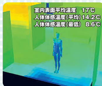
1枚ガラス(5ミリ)を使用した場合の室内表面温度分布
